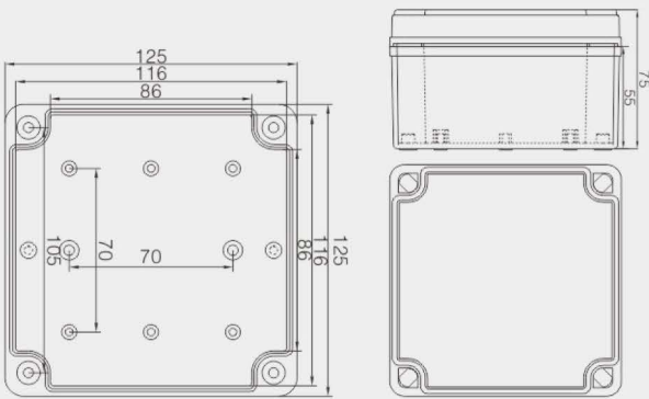
Outline dimension 外形尺寸图
