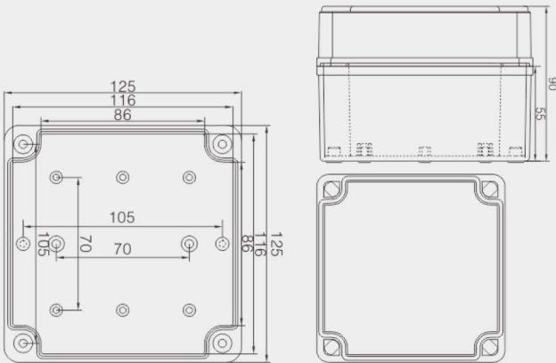
Outline dimension 外形尺寸图
