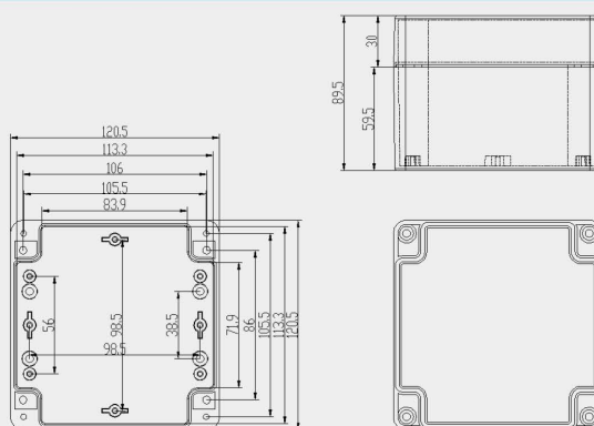
Outline dimension 外形尺寸图
